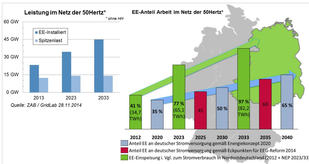
Abbildung 11.2-1: Installierte EE-Leistung im Netz der 50Hertz Transmission GmbH im Vergleich zur Spitzenlast und erwarteter Anteil EE-Anteil in diesem Übertragungsnetz
