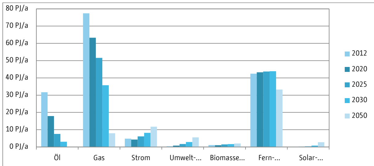
Abbildung 11.2-7: Endenergiemix für Heizung und Warmwasser im Handlungsfeld Gebäude
