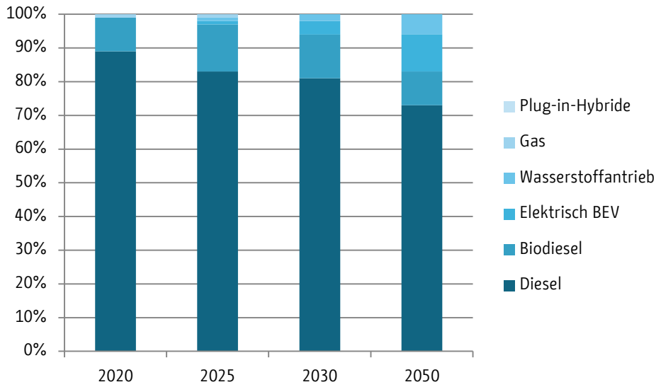
Abbildung 11.5-6: Flottenanteile 2020 – 2050 der schweren Nutzfahrzeuge bei Einsatz des Maßnahmenbündels
