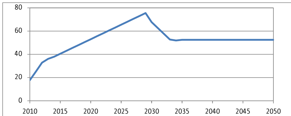
Abbildung 11.2-5: Installierte Photovoltaikleistung bei jährlichem Zubau von 2,5 GW p , 20 Jahren Lebensdauer
