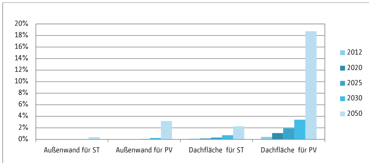
Abbildung 11.2-6: Flächenanteile Solare Nutzung
