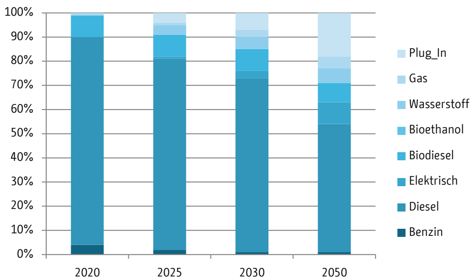
Abbildung 11.5-5: Flottenanteile 2020 – 2050 der leichten Nutzfahrzeuge bei Einsatz des Maßnahmenbündels
