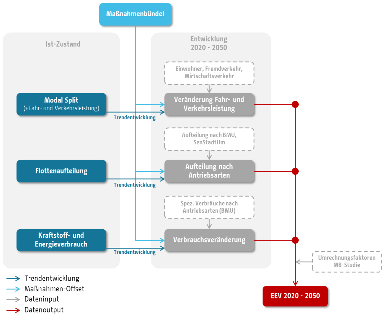
Abbildung 11.5-2: Ablaufschema für die verkehrliche Maßnahmenbewertung
