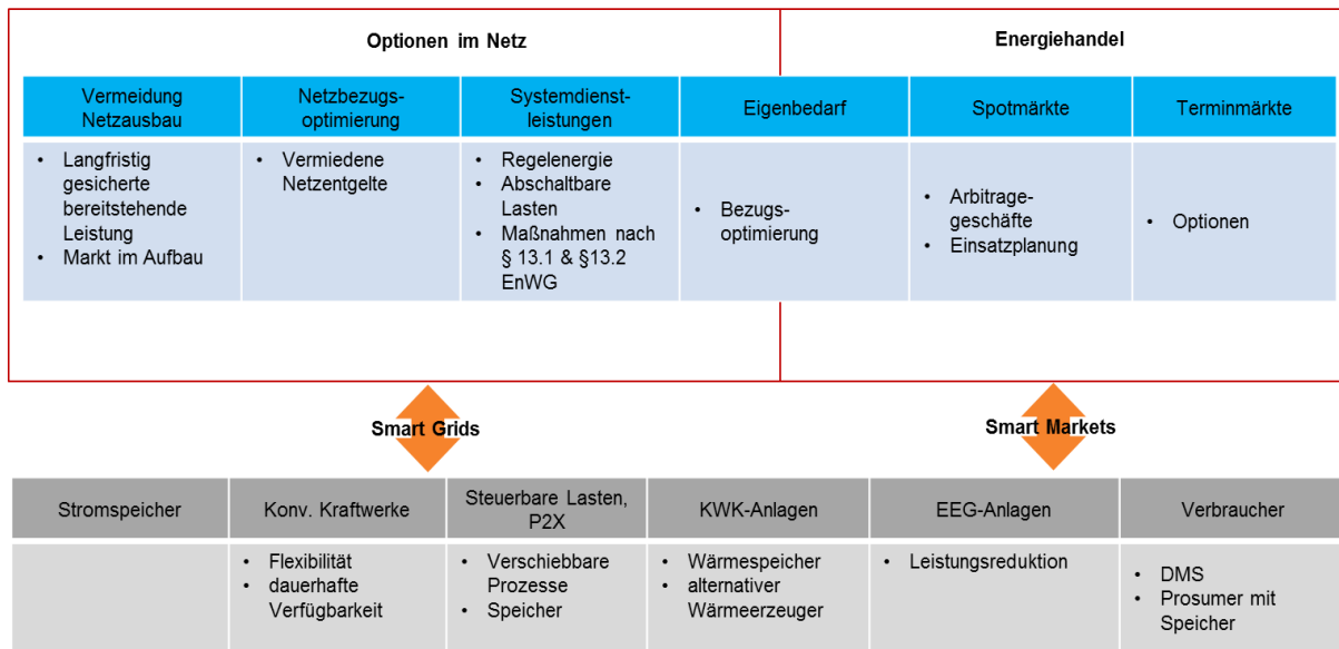
Abbildung 11.2-4: Märkte und Anbieter von Flexibilität
