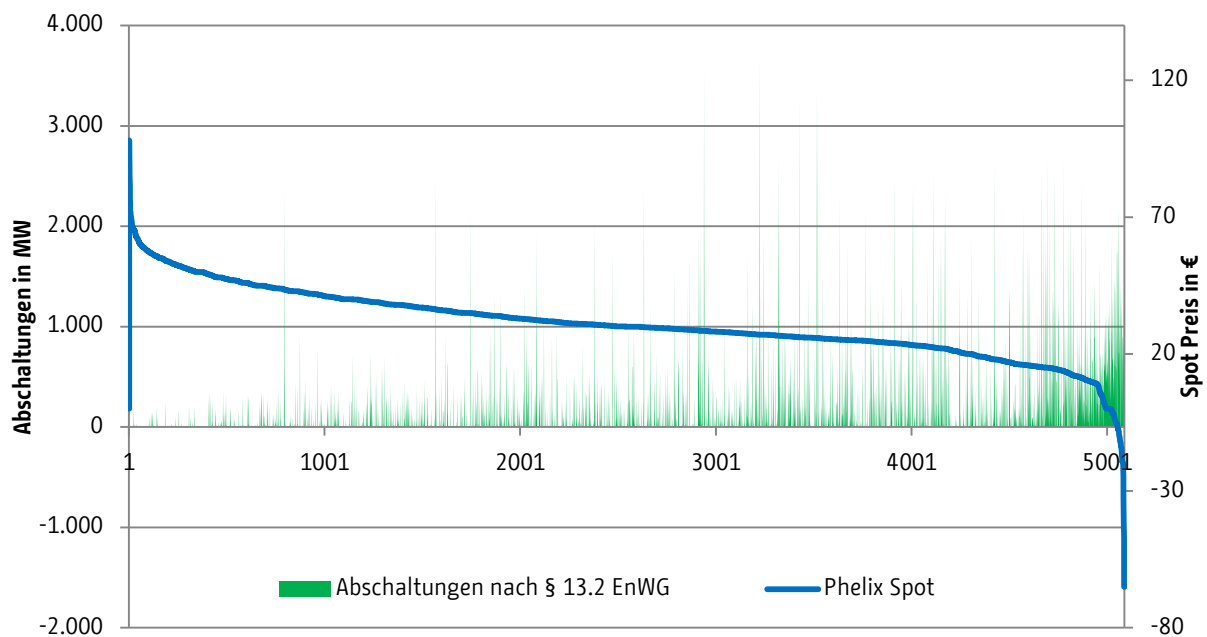
Abbildung 11.2-3: Geordnete Dauerlinie Spotpreis EPEX und zugehörige Abschaltungen nach § 13.2 EnWG bei der 50Hertz Transmission GmbH, Januar bis Juli 2015
