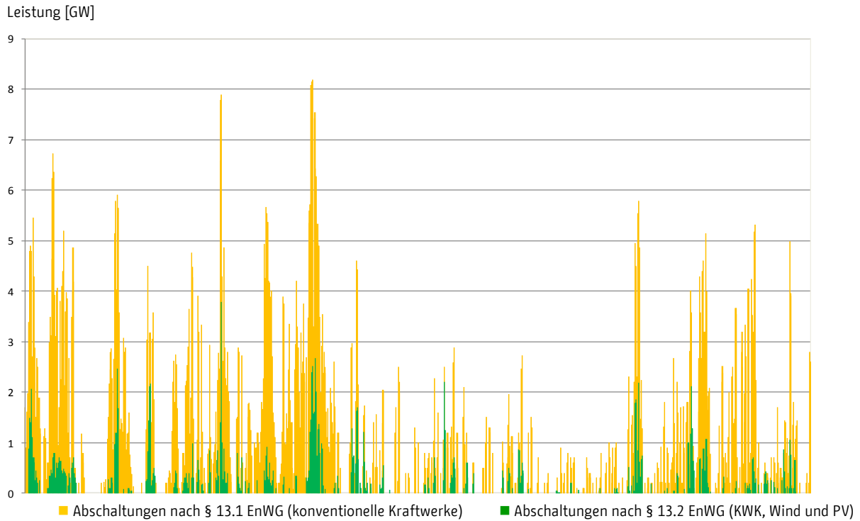
Abbildung 11.2-2: Abschaltungen nach § 13.1 und § 13.2 EnWG, Januar bis August 2015 im Netz der 50Hertz Transmission GmbH
